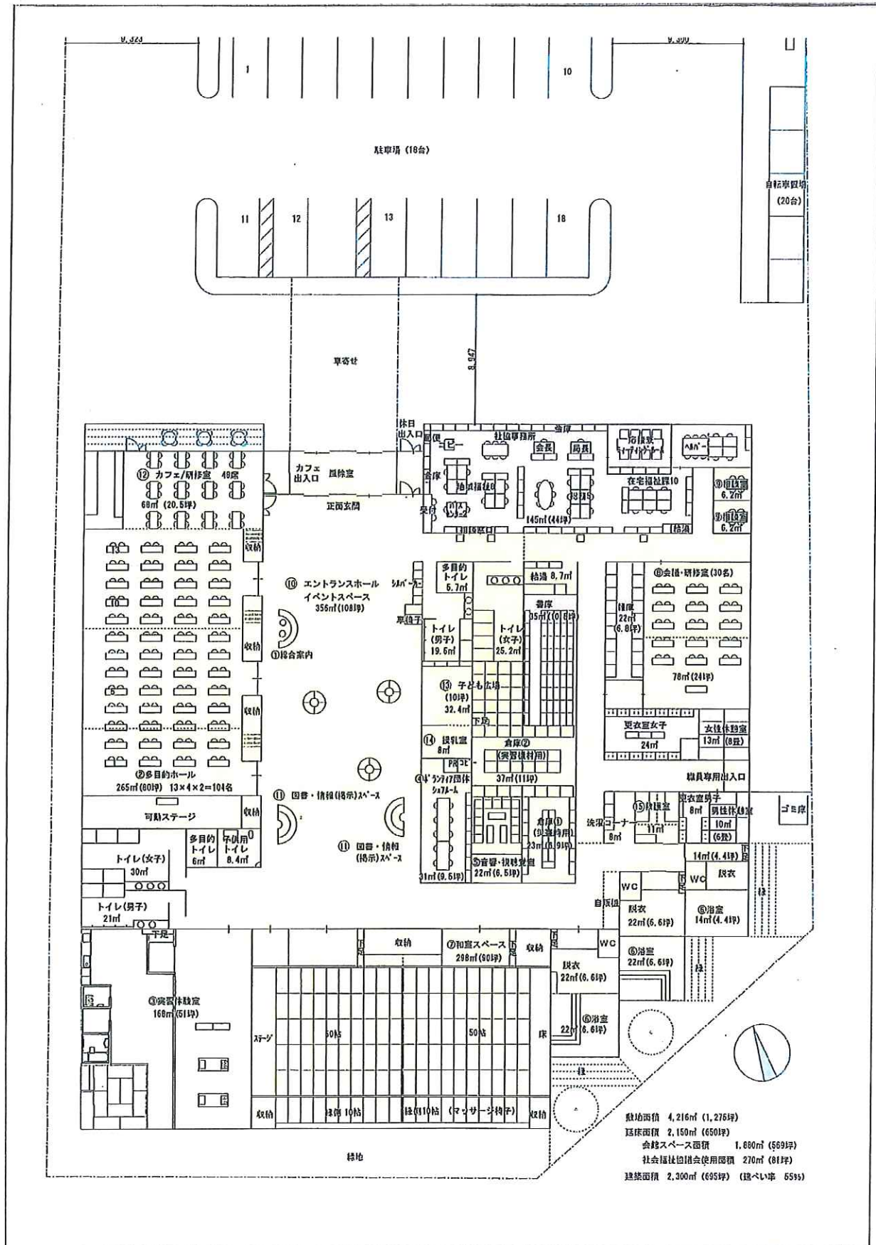
図 6-2 新総合福祉会館平面図
